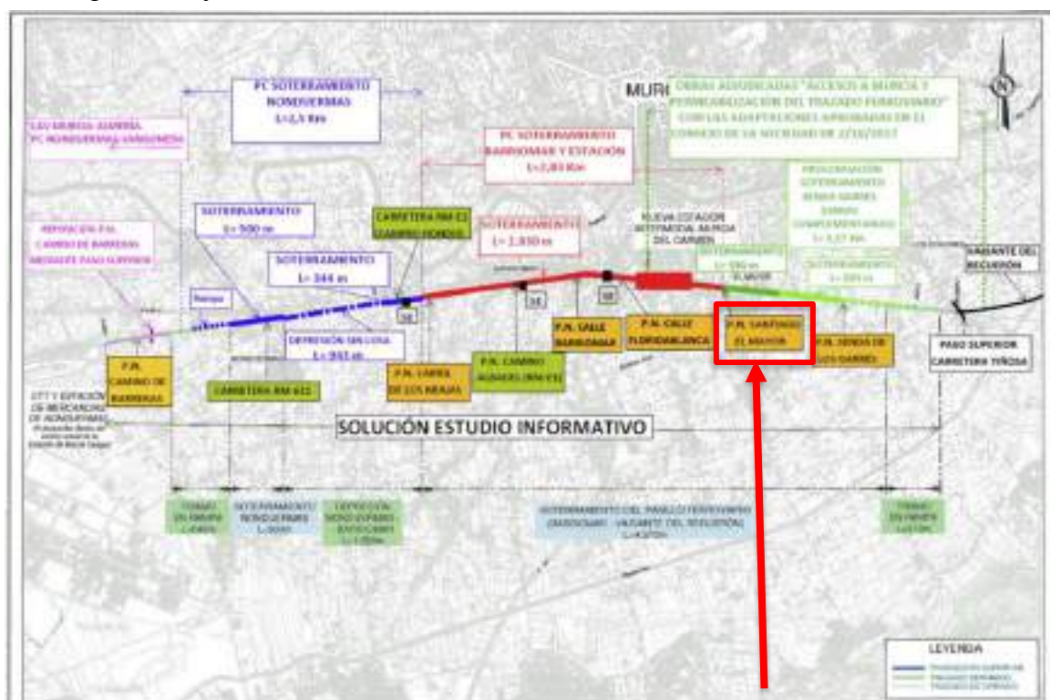
Plano de situación incluido en el ANEXO II de la resolución de 22 de mayo de 2019, relativo al soterramiento previsto al barrio de El Mayor en Murcia.-
